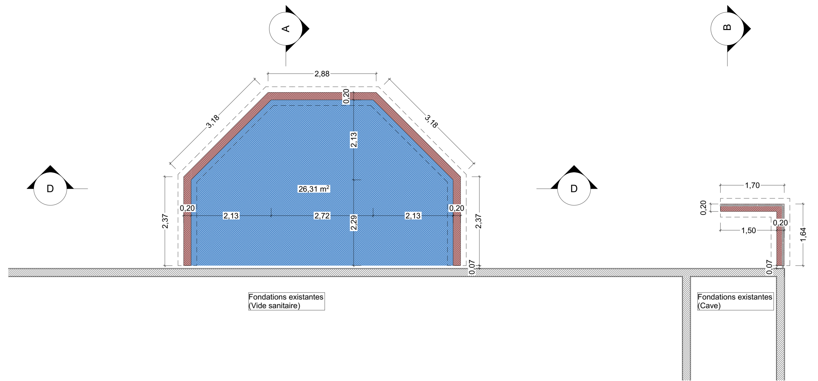
Fondations
